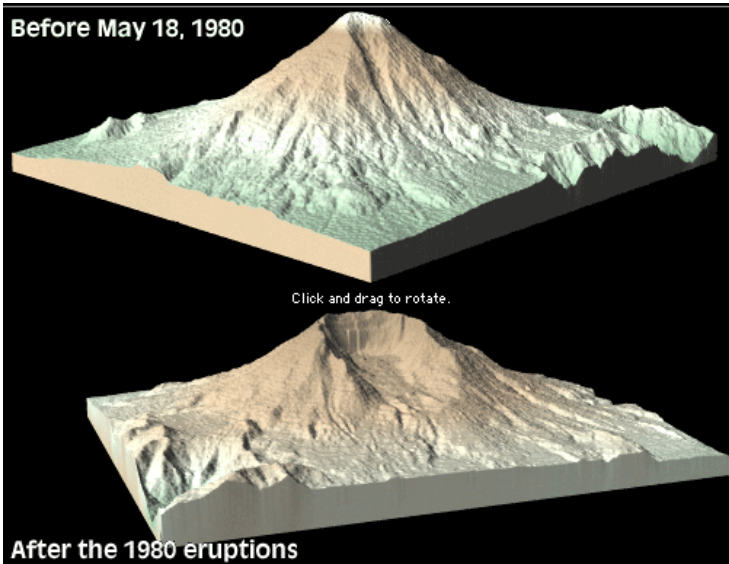
Monte Santa Helena - SE do Estado de Washington. Erupção de 1980. Típico arco vulcânico de margem continental
